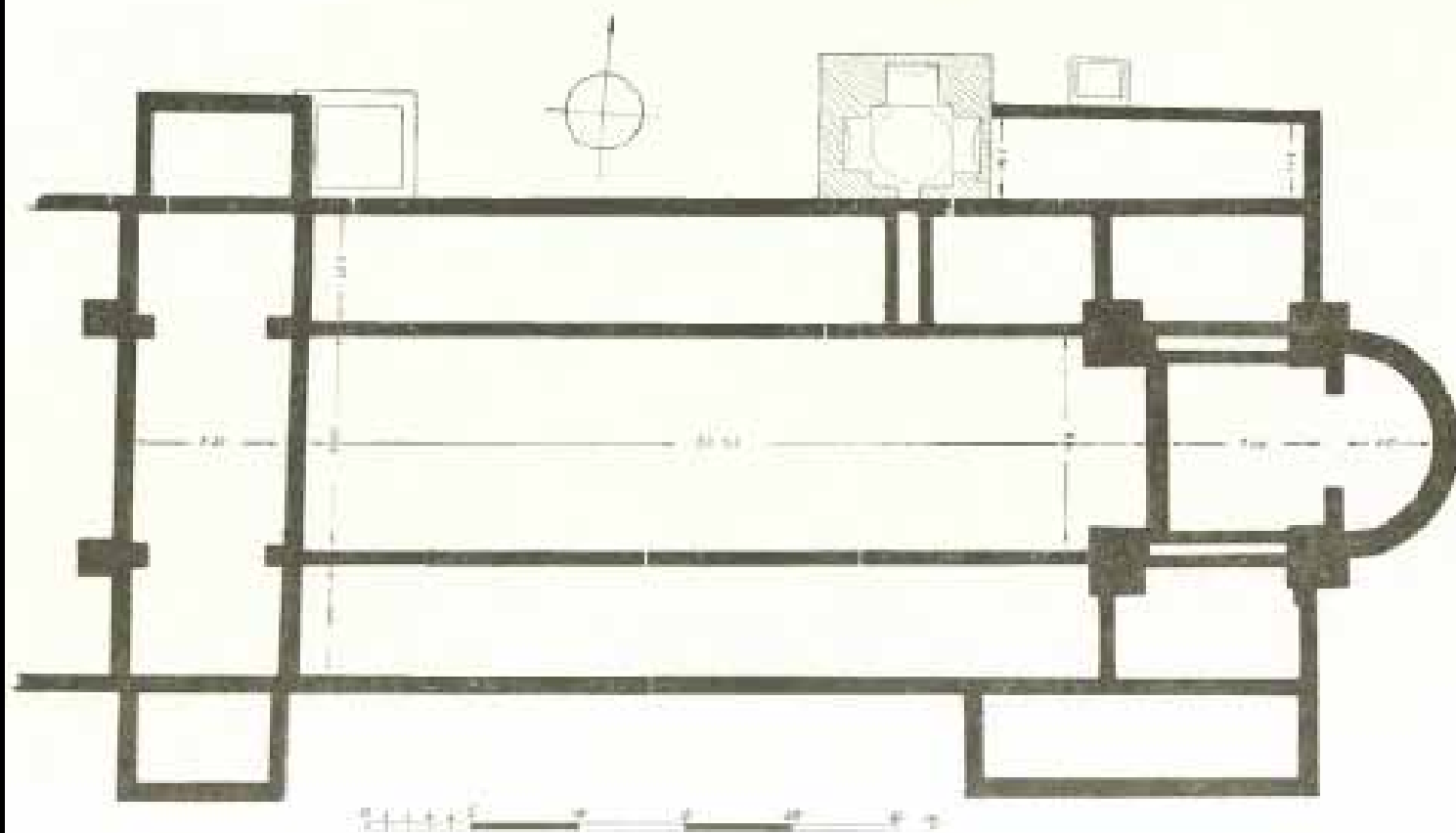
Εικό. 9. Κάτοψη των θεμελίων της βασιλικής (1948) συμπληρωμένη κατά την έκδοση ΑΕ 1919, εικό. 3, και Γ. Σωτηρίου, Χριστ. καὶ Θεζ. Ἀρχαϊκῶν, εικό. 189.
